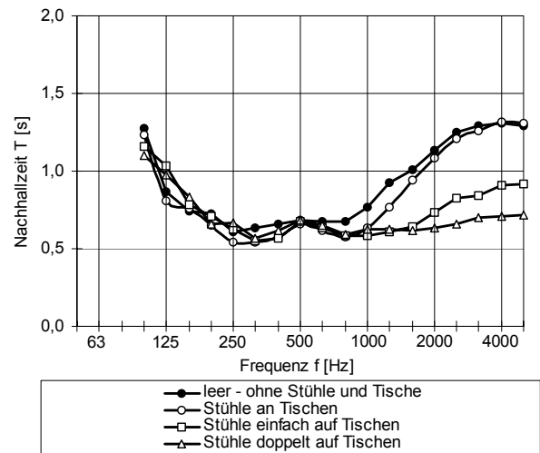
Abbildung 5: Messwerte der Nachhallzeiten in einem Unterrichtsraum mit massiven Innenwänden mit Deckensystem Typ 1 bei Variation der Diffusität
